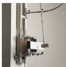
Attrezzatura per prova urti a temperatura ambiente.
