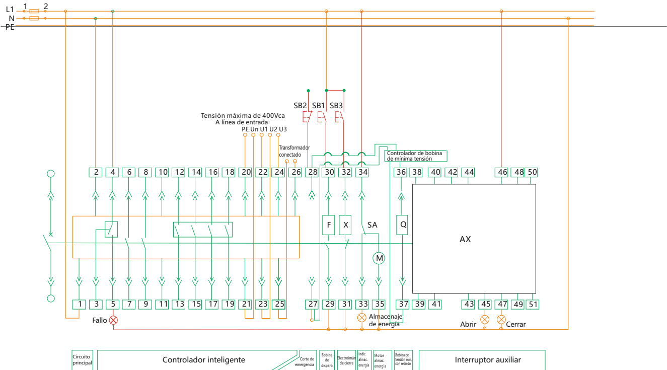
Cableado del circuito complementario para NA1-2000X~6300X con controlador inteligente tipo (3M) y bobina de mínima tensión con retardo
