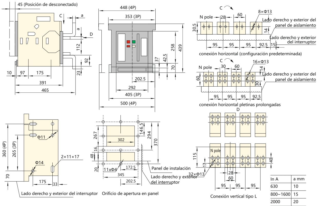
NA1-2000X/NA1-2000XN/NA1-2000XH Tipo extraíble, conexión posterior, vertical
