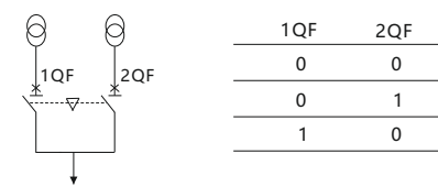
Esquema de circuito Modos de accionamiento disponibles
