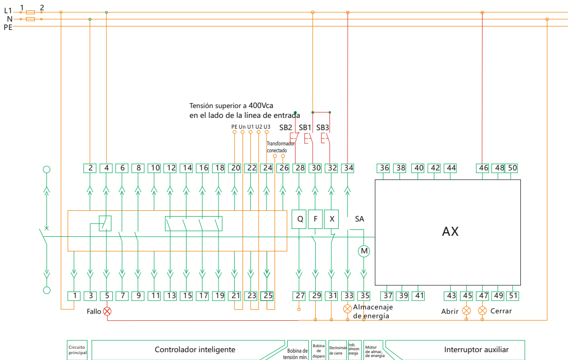
Cableado del circuito complementario para NA1-2000X~6300X con controlador inteligente tipo (3M) y bobina de mínima tensión instantánea
