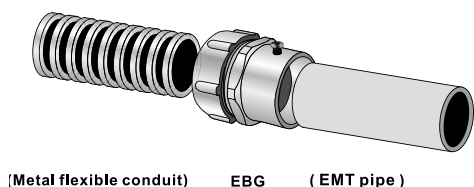
(Metal flexible conduit) EBG (EMT pipe)
